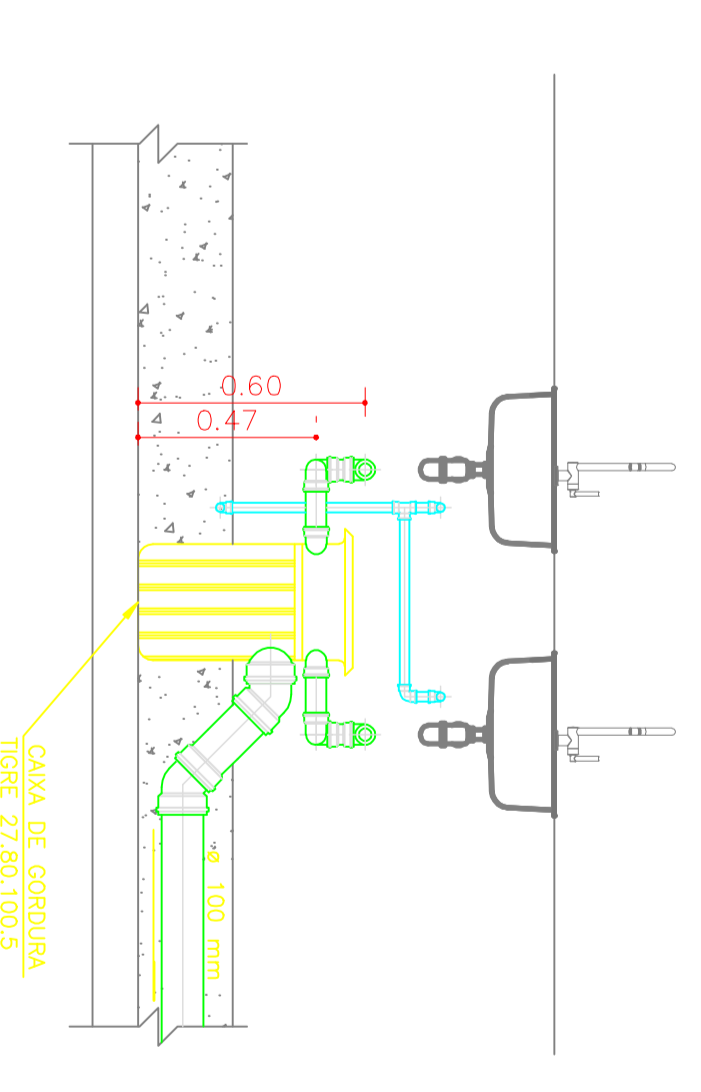
DETALHE PIA LANCHONETE - CAIXA DE CORDURA PAVIMENTO SUPERIOR ESC:1:20
